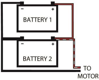
2 BATTERIES- 12 VOLT MOTOR
