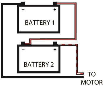
2 BATTERIES- 24 VOLT MOTOR
